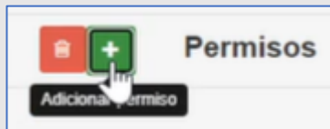
Ilustración 34: Adicionar Permisos
